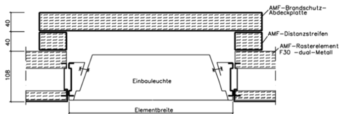
Bild 1 - Montagesatz für Bauseits gelieferte Leuchten
