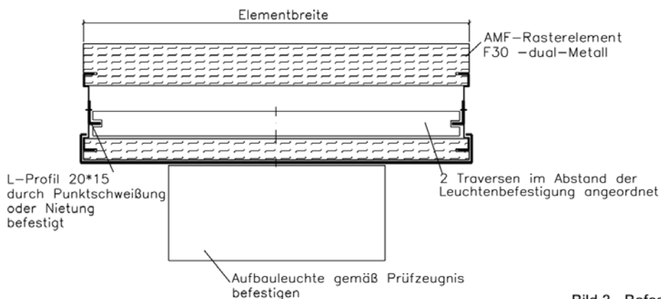
Bild 3 - Befestigungssatz für Aufbauleuchten
