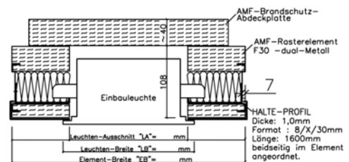
Bild 2 - Befestigungssatz werkseitig im Element montiert für bauseits zu montierende Einbauleuchten
