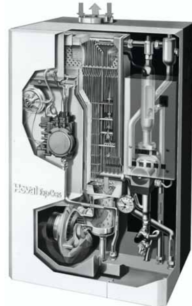
Schnittbild TopGas M condens ohne Pumpe
